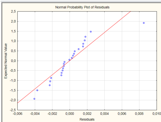
Фиг.10. Нормална вероятностна графика на остатъците на модела (3) за параметър y_1
