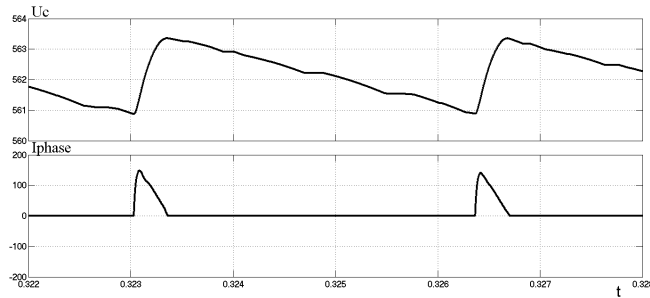
Фиг. 22. Напрежение на кондензатора и мрежов ток
