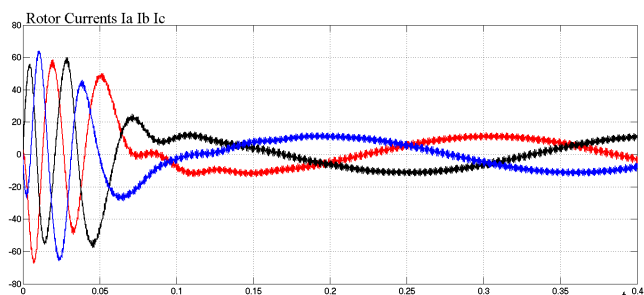
Фиг. 9. Роторни токове
