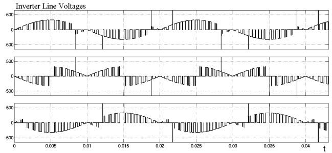
Фиг. 24. Линейни напрежения на инвертора при използване на еднофазен двуполупериоден мостов изправител (схема Грең) без включен капацитивен филтър
