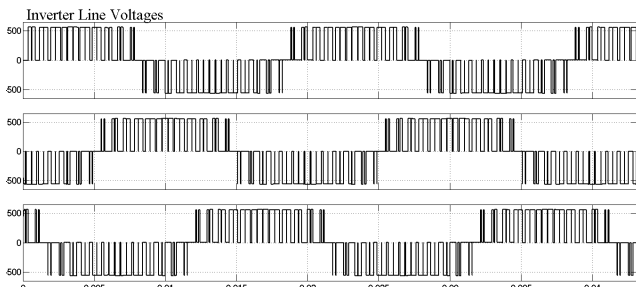
Фиг. 7. Линейни напрежения на инвертора
