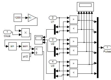
Фиг. 4. Структурна схема за получаване на управляващи импулси
